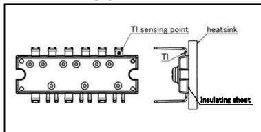
TI sensing point
